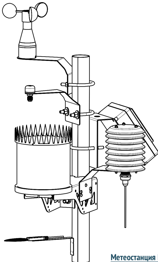
Рис.1 Метеостанция Kairos
