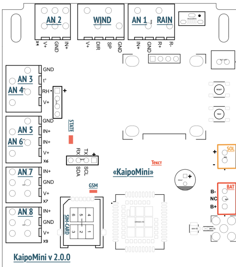
Рис. 5 Схема подключения датчиков к станции
